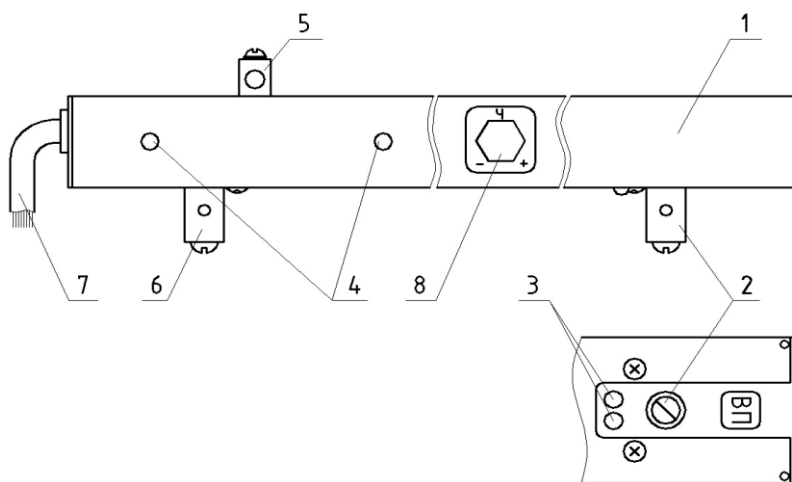
Рисунок 1.3 Конструкция ПРМ.
